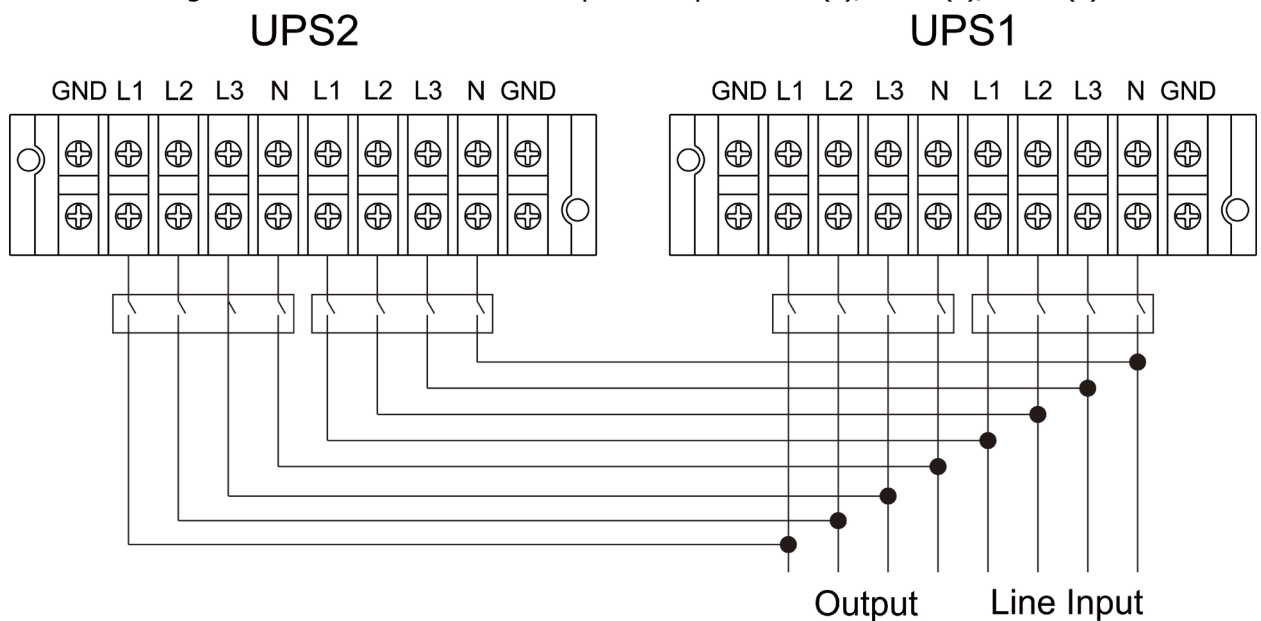
Figura connessioni del sistema parallelo per 30000(L)
